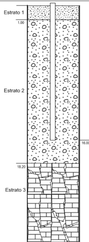
Figura 1. Esquema de la estratigrafía considerada para la solución de pilotes flotantes.
