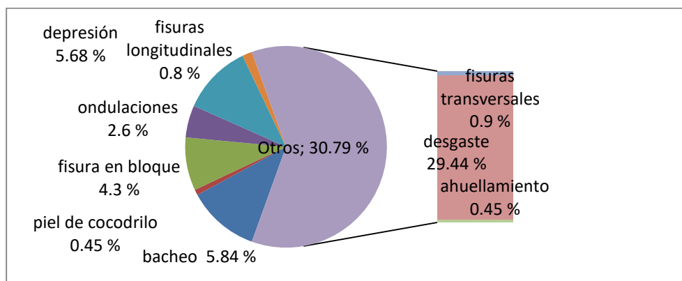
Figura 4. Mayores desperfectos encontrados en el carril izquierdo
