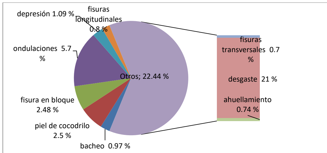
Figura 5. Mayores desperfectos encontrados en el carril derecho
