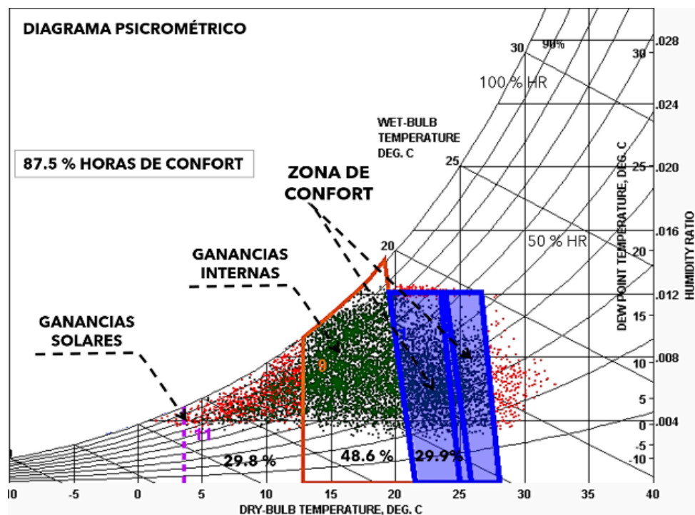
Figura 4. Carta psicrométrica de Givoni. Fuente: Generada en Climate Consultant, modelo de confort ASHRAE 55.
