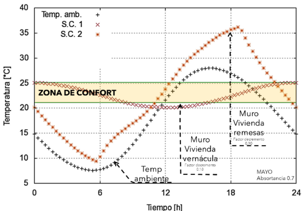
Figura 7. Comparación de la envolvente de la VT y VR. Fuente: simulación generada en Ener Habitat.
