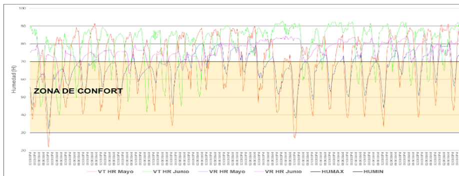
Figura 6. Humedad relativa en VT y VR en mayo-junio 2021. Fuente: Elaboración propia con datos de HOBOware.
