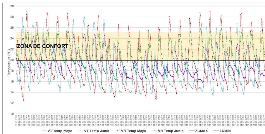
Figura 5. Temperaturas de VT y VR en mayo-junio 2021. Fuente: Elaboración propia con datos de HOBOware.
